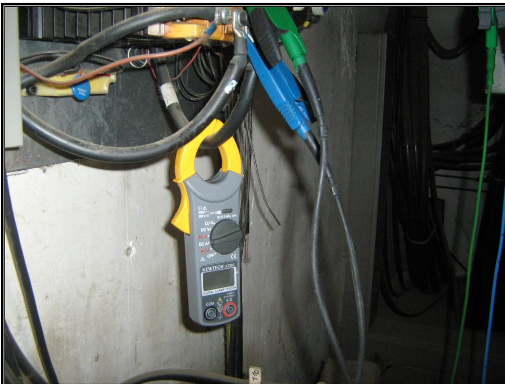
Imatge de l'amperímetre. Ens permet anotar els valors corresponents a la intensitat d'excitació de l'assaig. L'amperímetre està acoblat, com es pot veure a la foto, per mitjà d'una pinça que li permet aconseguir les dades corresponents.
