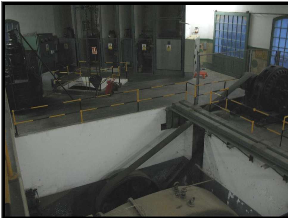
Imatge aèria de la central realitzada des del punt on hi ha la sala i l'ordinador de control. S'hi poden observar 2 de les 3 turbines (L'altre, la 3, està a una sala contigua), un generador, i els transformadors. (Imatges d'elaboració pròpia)
