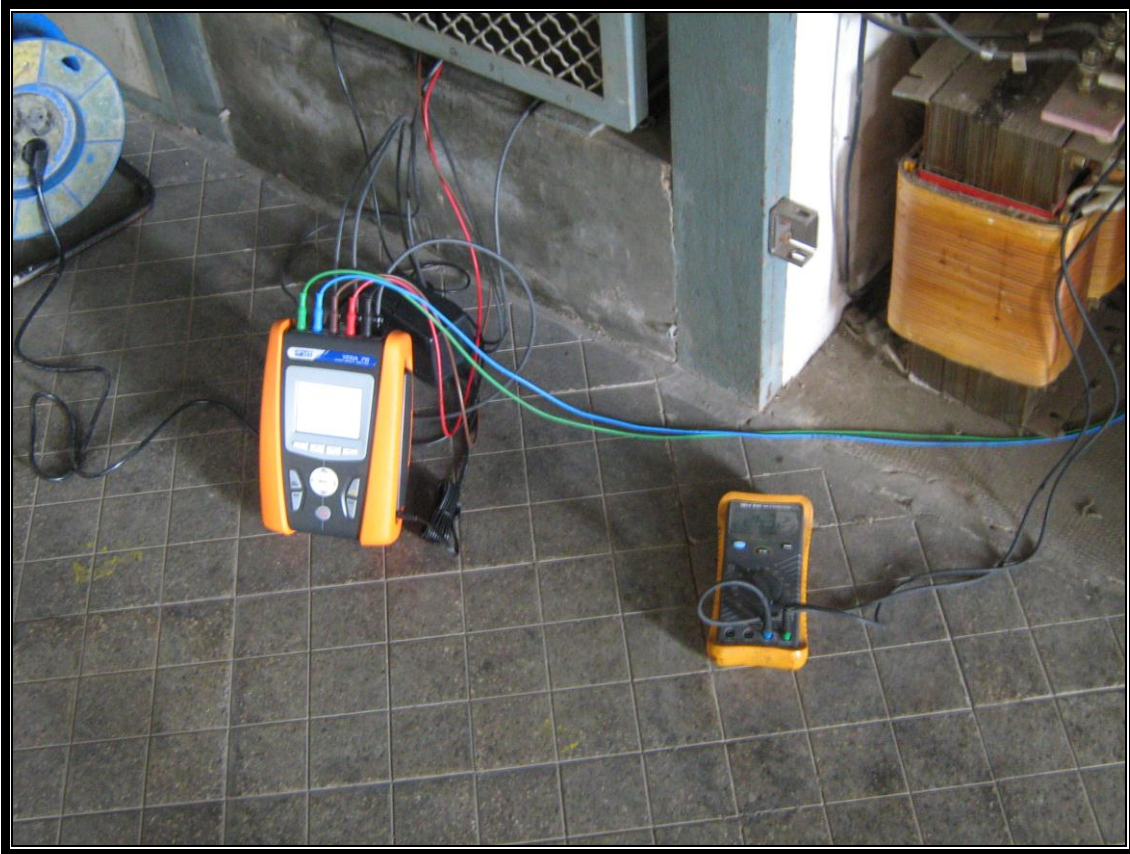
Fotografia del muntatge en conjunt al transformador de la central. A l'esquerra, el panell electrònic. A la dreta, el voltímetre.
